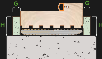
Marco para Jamba Recta
